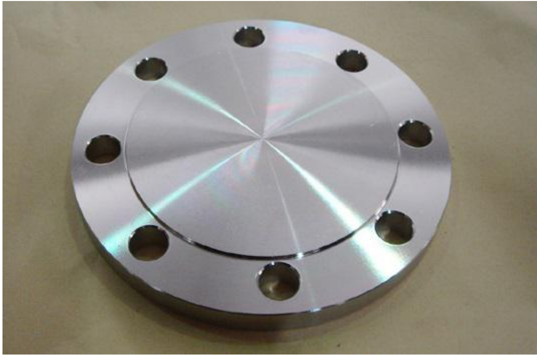
上图为 ANSI 2500LB BL 盲板法兰或近似法兰
